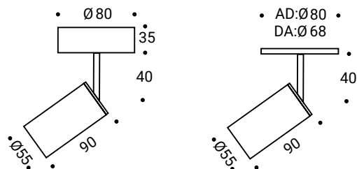
Maße (mm)
